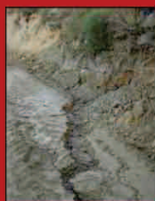
Día 3 de septiembre de 2008. Primer llenado de la balsa y primeras fugas
